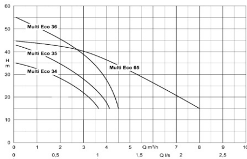
Multi-Eco P modelo portátil (<14 kg)
